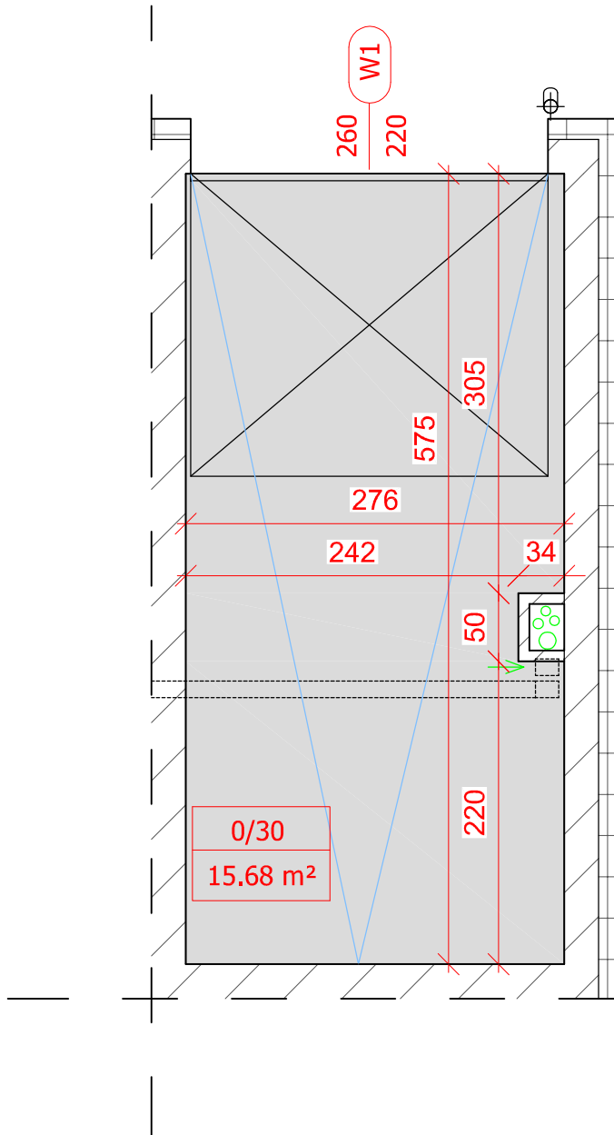
Rzut garażu skala 1:50
